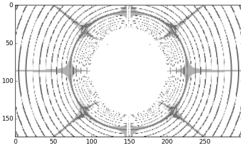
Schwarzschild ( m=0.3 )
