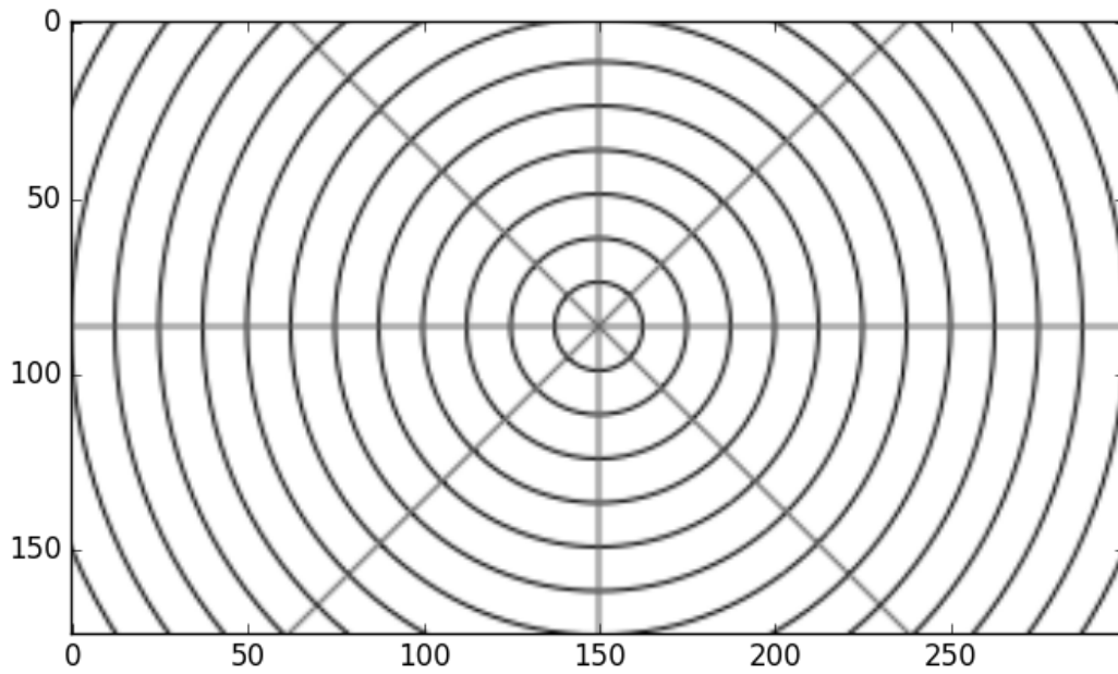
No lensing (Minkowski)
